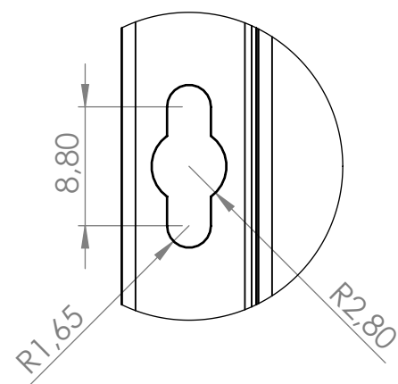
DÉTAIL A ECHELLE 2 : 1
